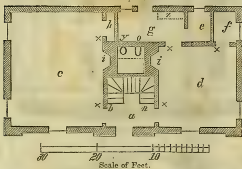
Fig. 23. Ground-plan.
